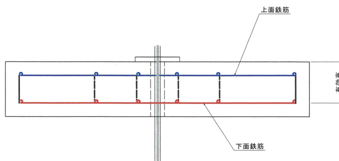
【標準配筋図】
